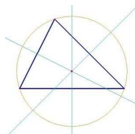
Las mediatrices de un triángulo se cortan en el circuncentro.
