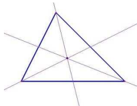
Las medianas de un triángulo se cortan en el baricentro.
