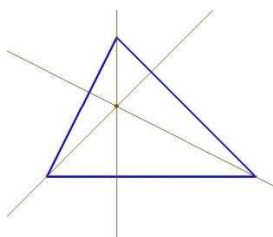
Las alturas de un triángulo se cortan en el ortocentro.
