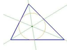
Las bisectrices de un triángulo se cortan en el incentro.
